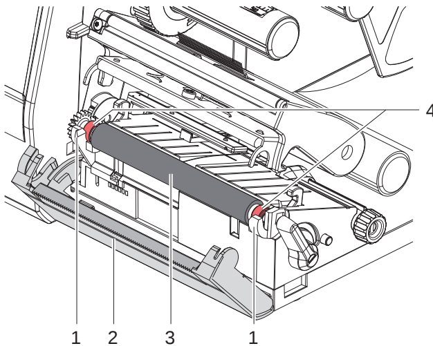
Figura 15 Rodillo de presión
