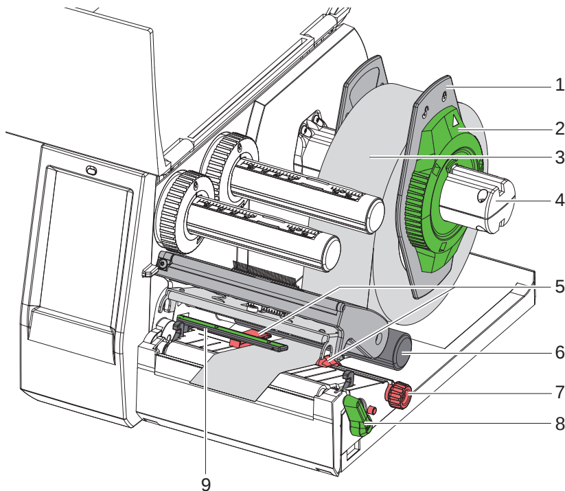
Figura 9 Colocación del material en carrete
