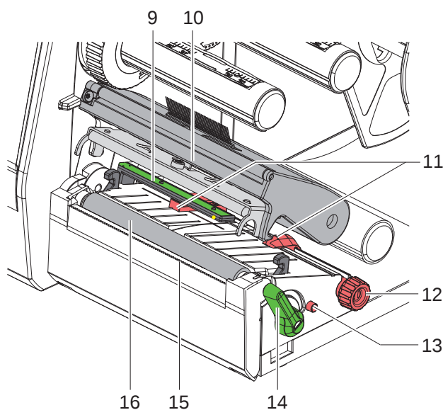
Figure 2 Mécanisme d'impression
