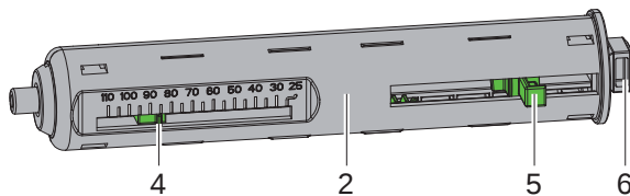
Bild 18 Transferfolienkern anpassen
