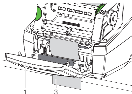
Bild 14 Etiketten für Spendemodus einlegen
