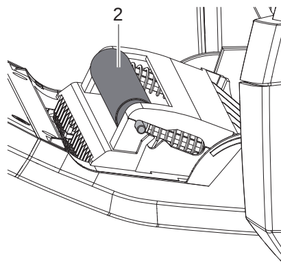
Andruckwalze in Arbeitsposition
