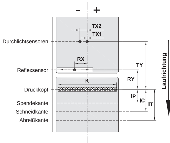
Bild 24 Gerätemaße
