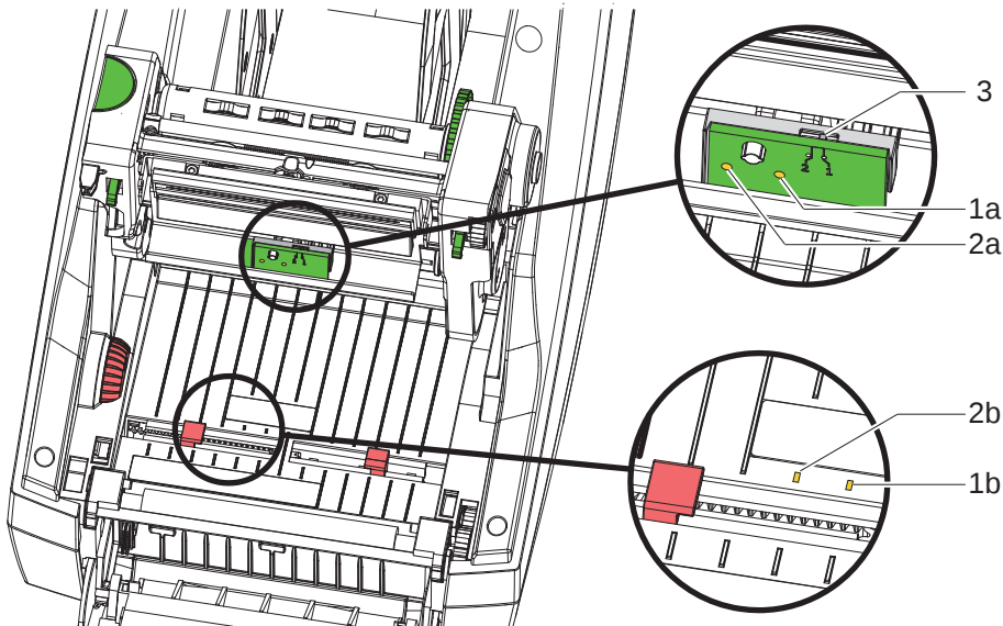
Bild 15 Durchlichtsensor auswählen
