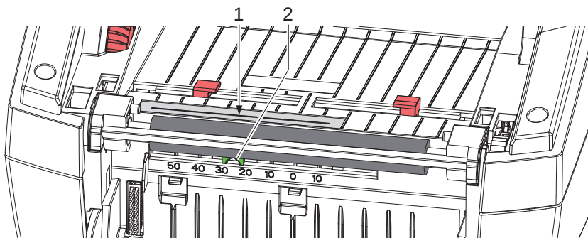
Bild 16 Reflexsensor positionieren
