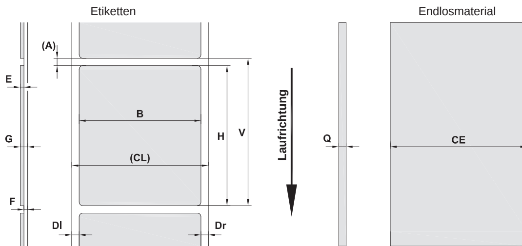
Bild 23 Maße Etiketten / Endlosmaterial
