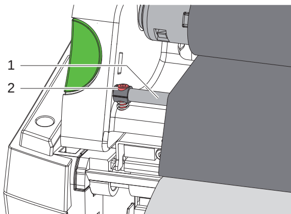
Bild 20 Transferfolienlauf einstellen
