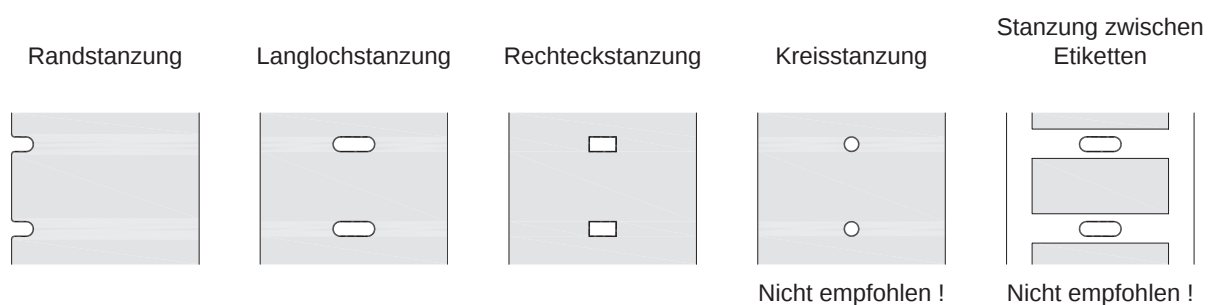
Bild 27 Beispiele für Stanzungen
