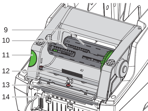
Bild 2 Druckmodul
