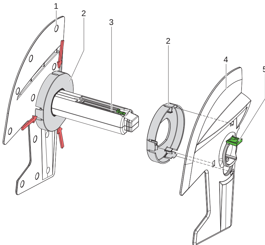
Bild 9 Rollenaufnahme anpassen
