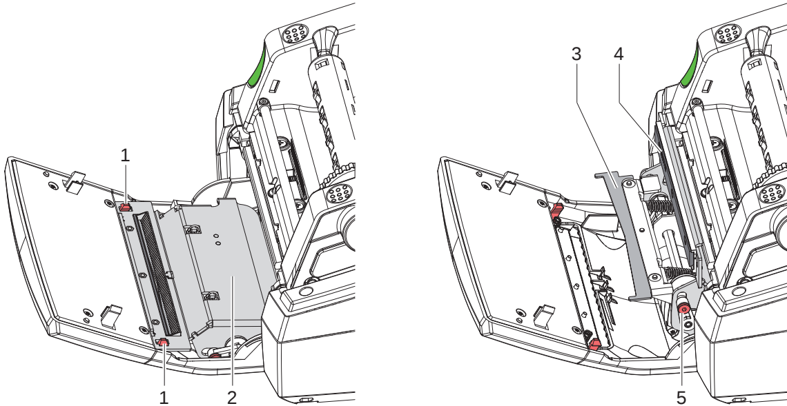
Bild 21 Messer reinigen
