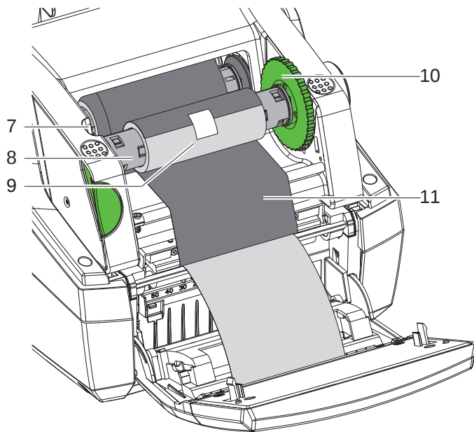
Bild 19 Einlegen der Transferfolie
