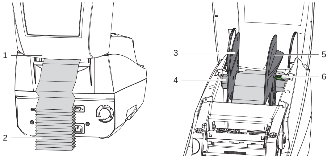
Bild 12 Leporello-Etiketten einlegen
