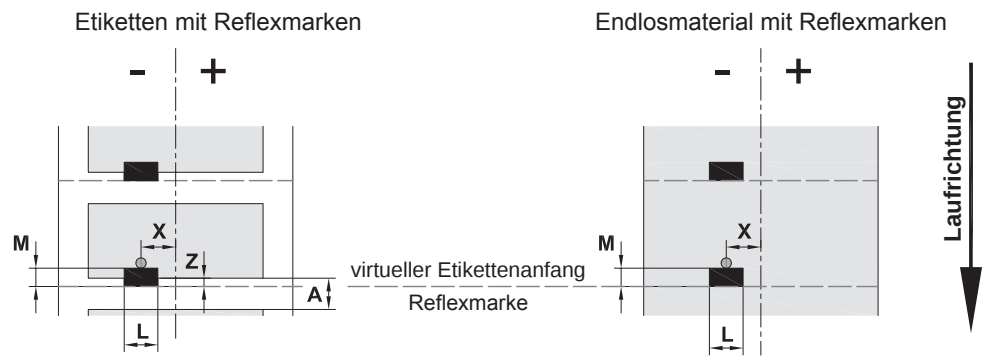
Bild 25 Maße für Reflexmarken
