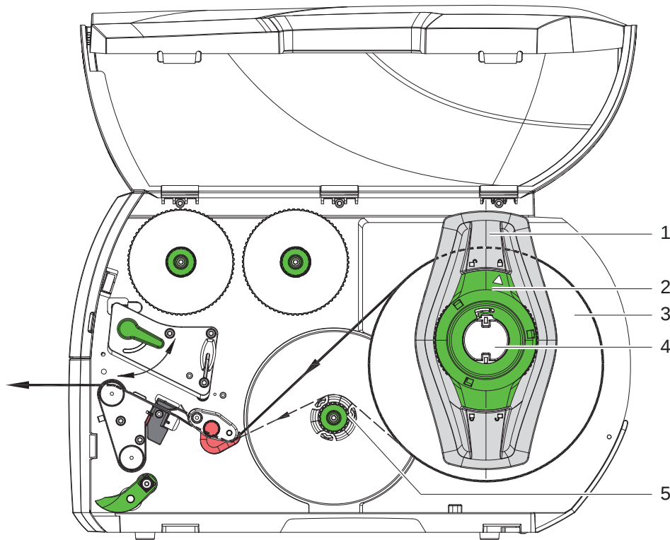
Afbeelding 12 Rolmateriaal invoeren
