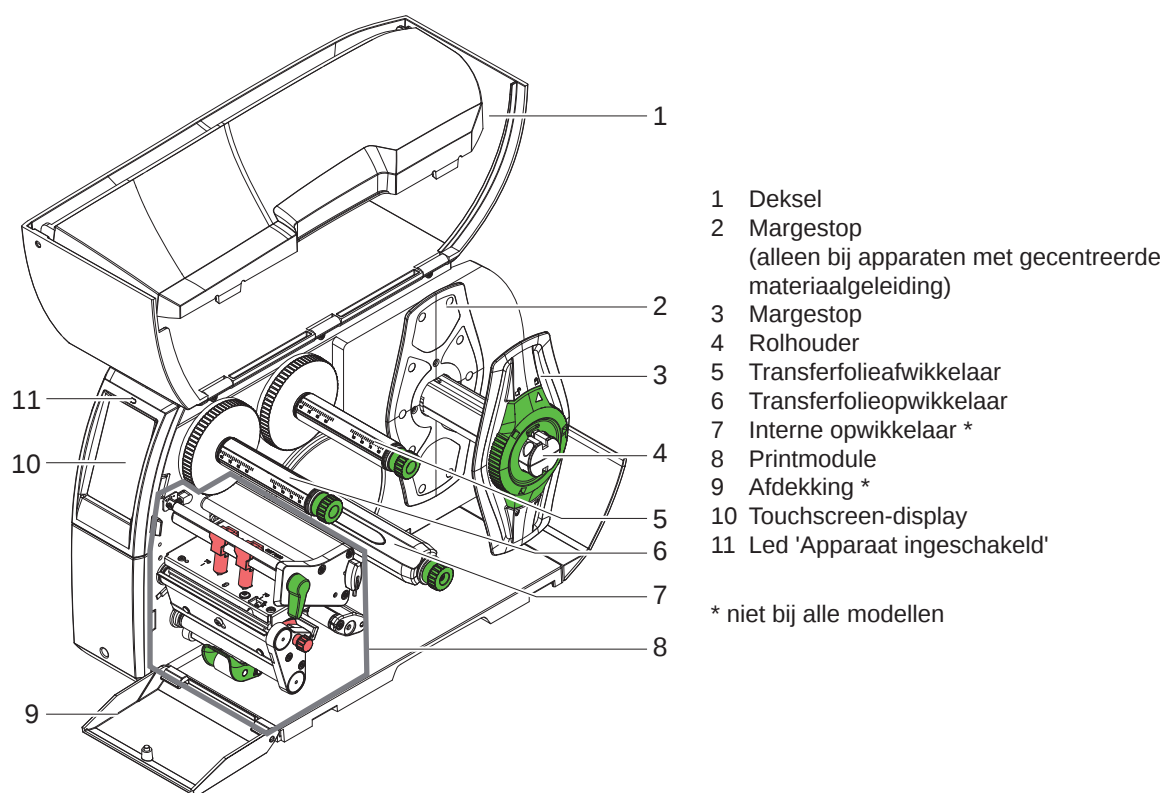
Afbeelding 1 Overzicht
