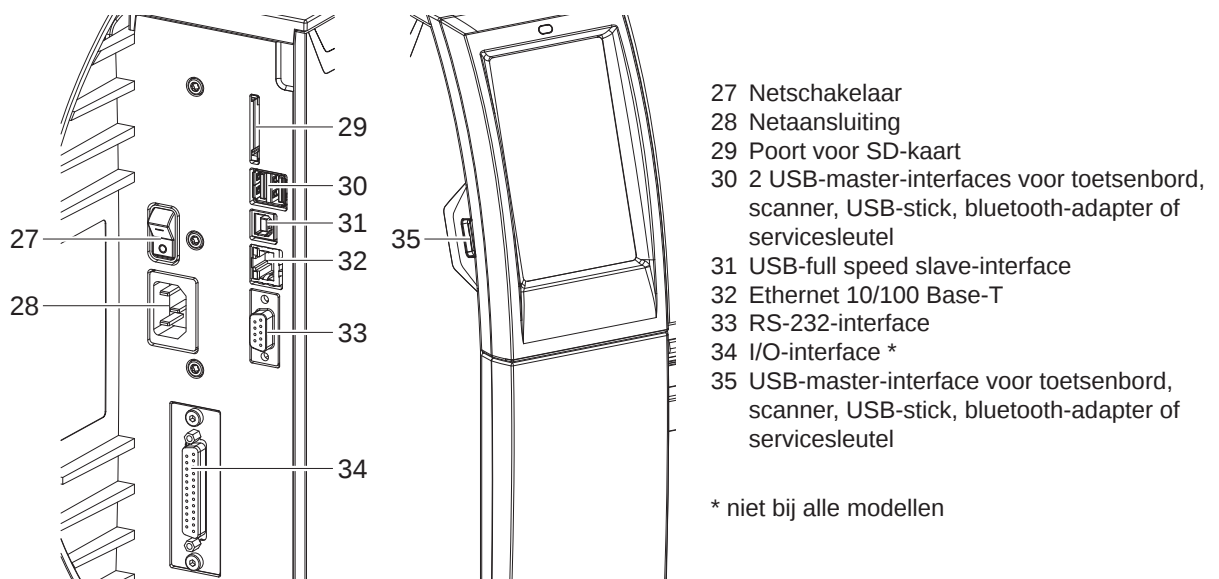
Afbeelding 5 Aansluitingen
