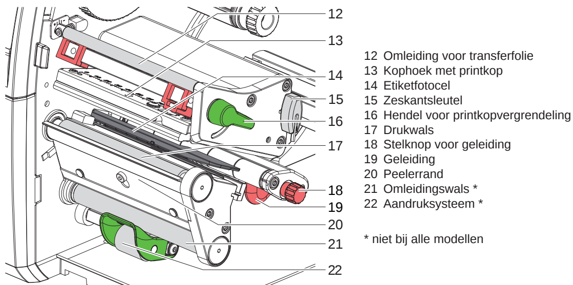
Afbeelding 2 Printmodule - apparaten met links uitgelijnde materiaalgeleiding
