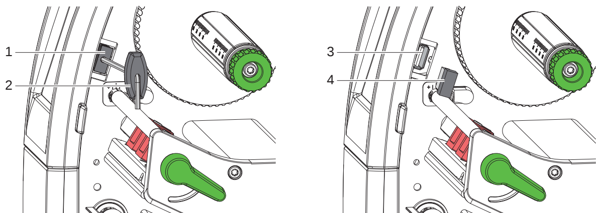
Afbeelding 6 Wifi-stick installeren
